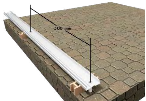
8. Separación entre tornillos rastrel.
