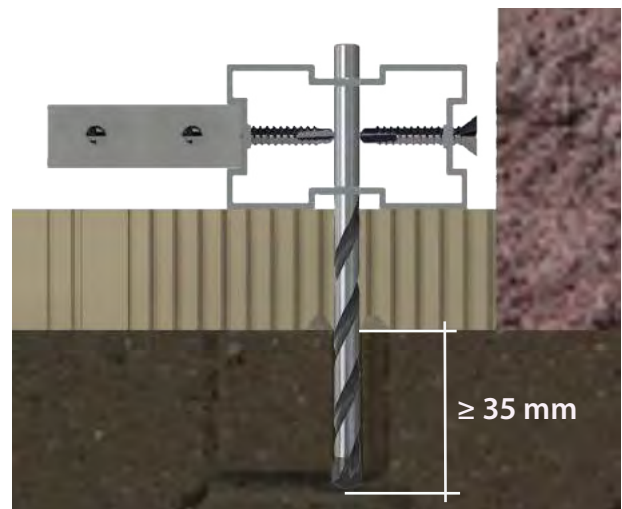
28. Taladro del suelo con broca de hormigón.
