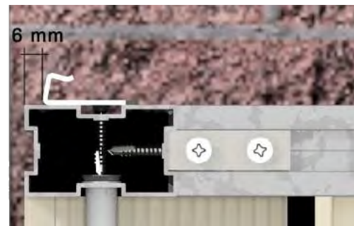
34. Detalle vista lateral clip de inicio
