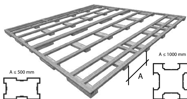
14. Luz máxima separación losetas. según tipo de rastrel.
