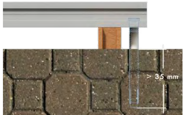
7. Distancia mínima penetra tornillo en suelo.
