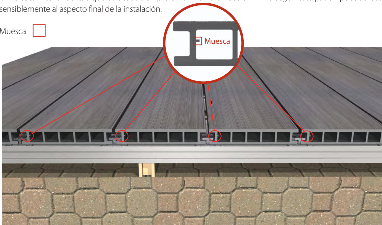
43. Colocación correcta dirección muescas
