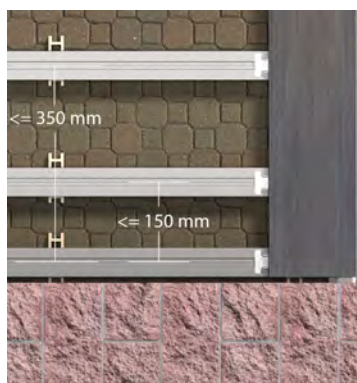
20. Distancias entre rastreles en extremos
