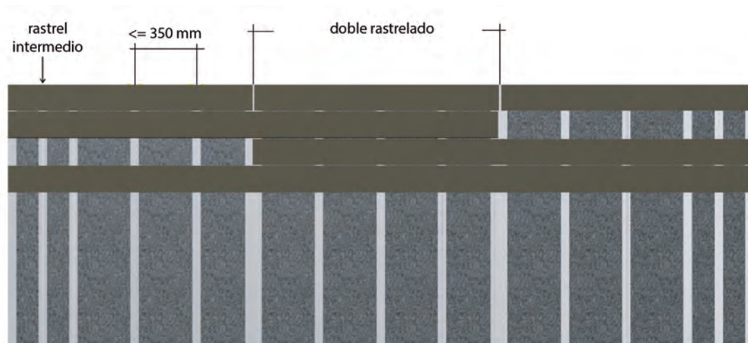
22. Rastrelado con lamas de distintas longitudes.
