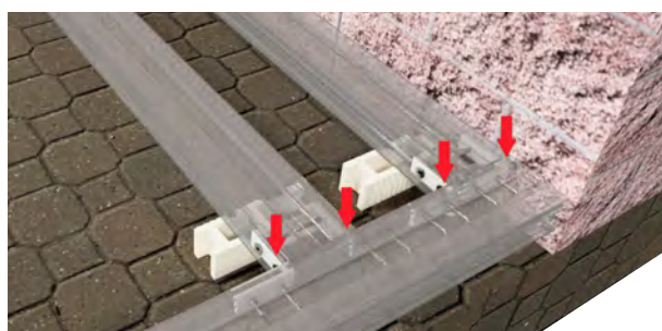
31. Vista de las escuadras perimetrales fijada al rastrel longitudinal perimetral.
