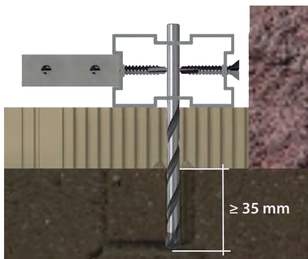
28. Taladro del suelo con broca de hormigón.
